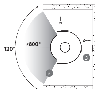
DISTANCES DE SÉCURITÉ
