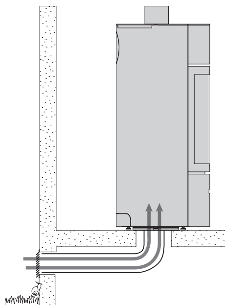
arrivée d'air sous le foyer
