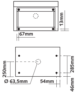
BOVENAANZICHT
