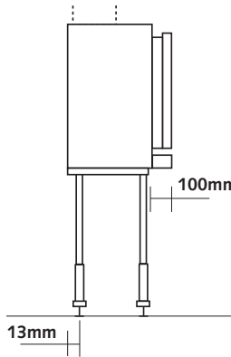
ZIJAAANZICHT
