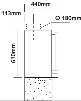
ZIJAAANZICHT
