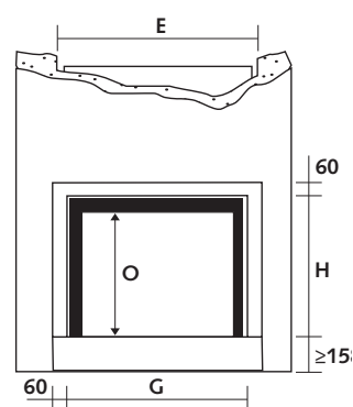
Te voorziene reserve bij plaatsing van een kader met tegenkader stuv (afwerking met kader stuv).
