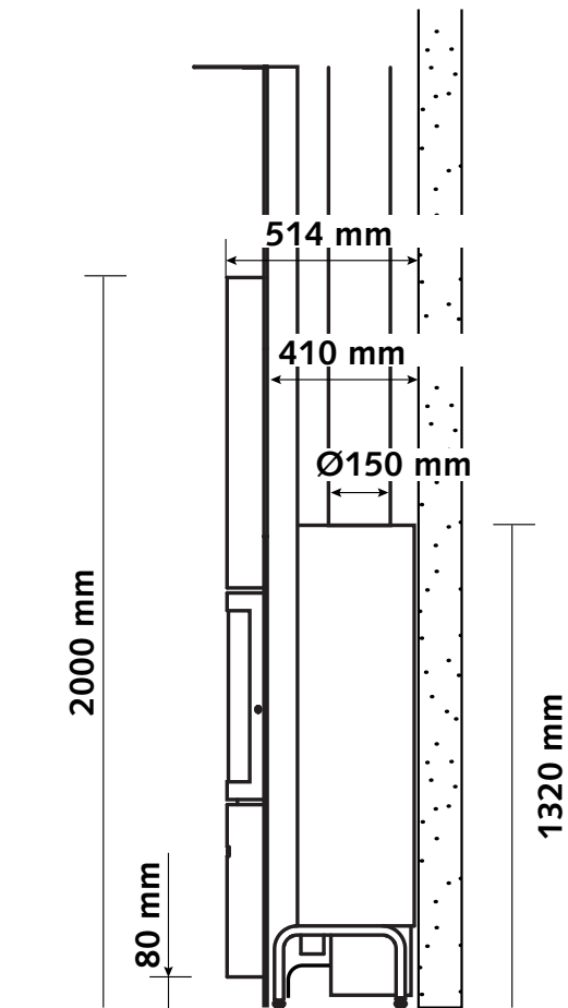
SEITENANSICHT
