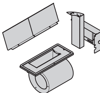
VENTILATOR-BAUSATZ
