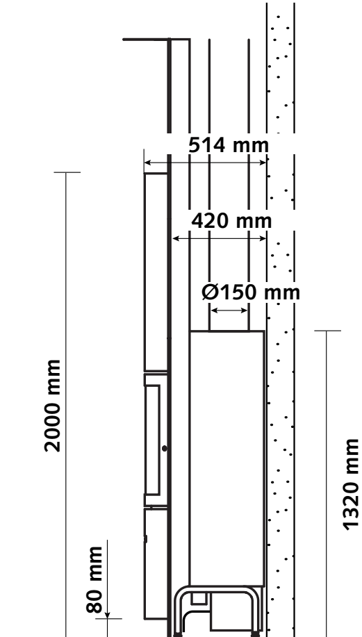
SEITENANSICHT
