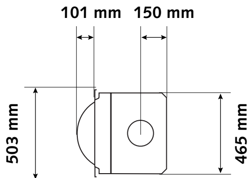
DRAUFSICHT
