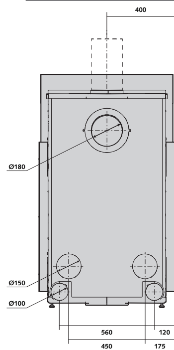
ACHTERAANZICHT
