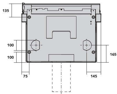
ONDERAANZICHT
