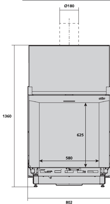
VOORAANZICHT
