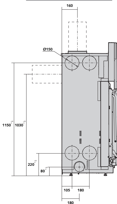
ZIJAAANZICHT
